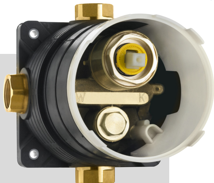
Keramická hlavica
