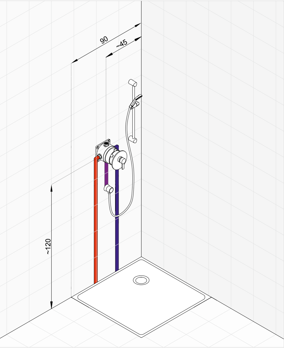
Klasický podomietkový rozvod k sprchovej zostave.
