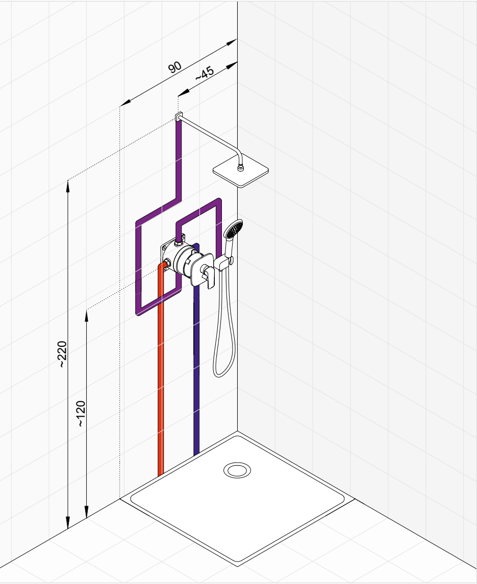
Klasická kombinácia podomietkovej batérie pre hlavovú a ručnú sprchu. Získame dva zdroje vody, všetko je riadené jednou podomietkovou batériou s prepínačom.
