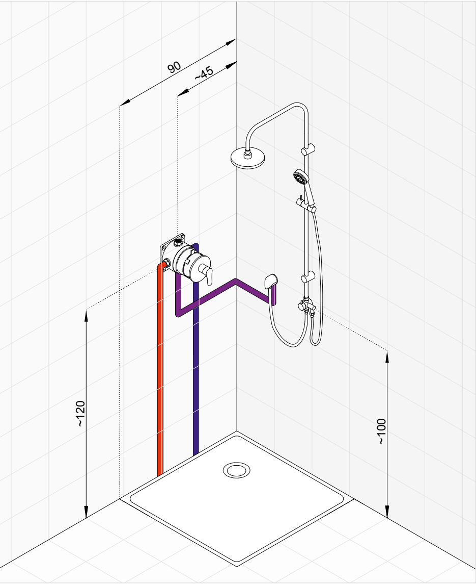
Zostava KLUDI DUAL SHOWER SYSTEM ponúka ručnú a hlavovú sprchu integrovanú do jedného setu. Voda je dodávaná jednou podomietkovou vodnou cestou do hadicovej prípojky.
