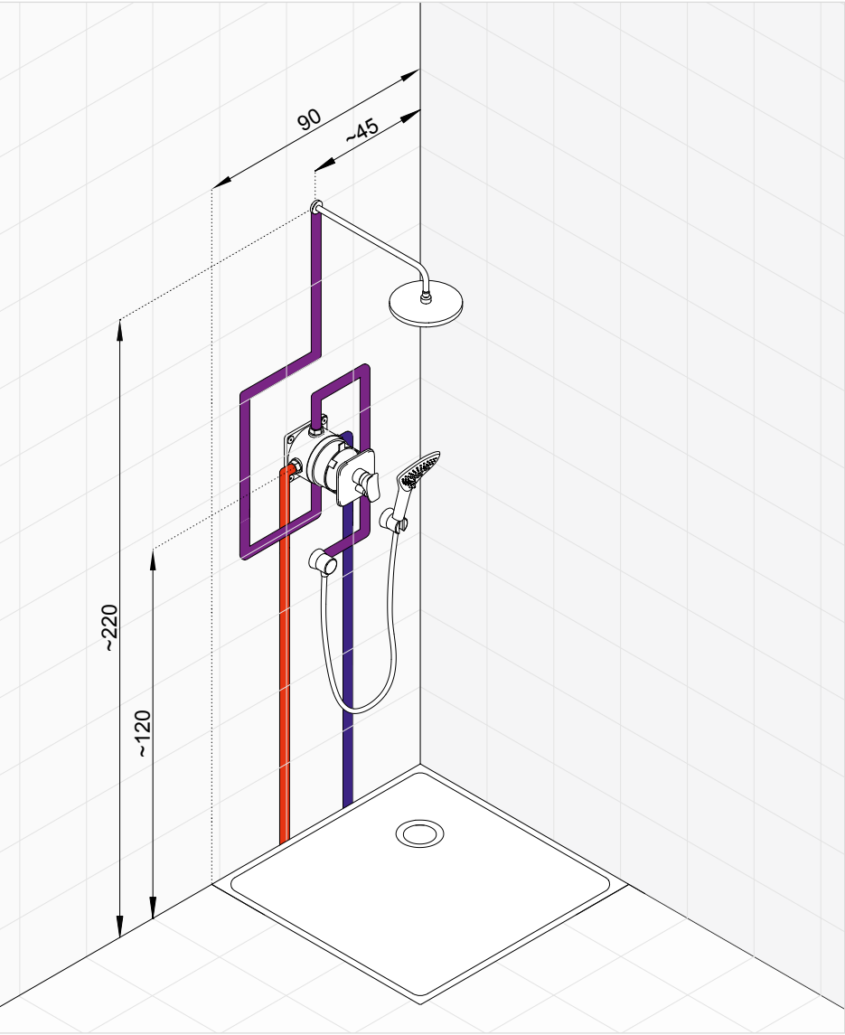
Klasická zostava podomietkovej batérie pre hlavovú a ručnú sprchu. Získame dva sprchové vývody vody a všetko je ovládané jednou podomietkovú batériou s prepínačom.
