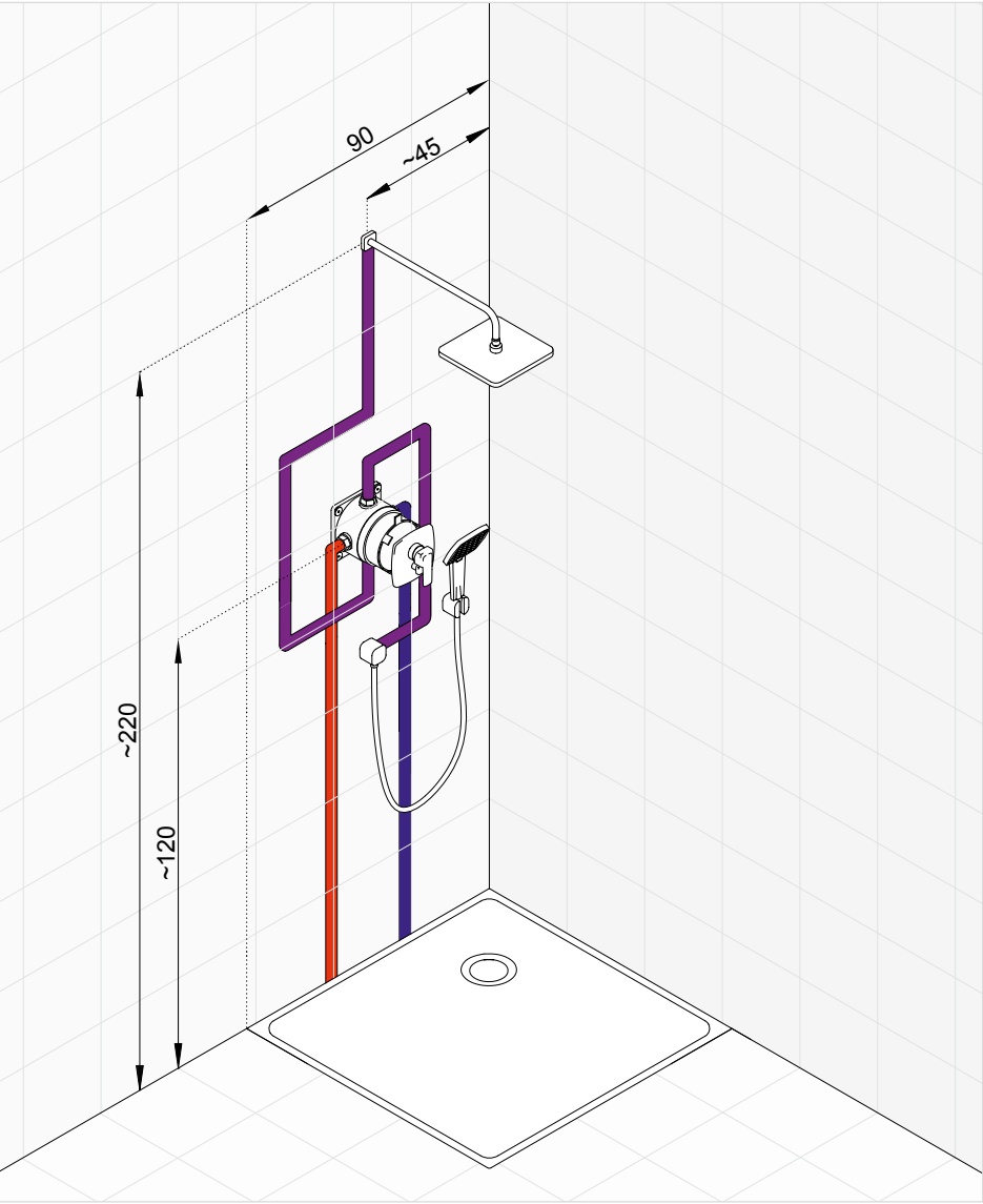
Klasická zostava podomietkovej batérie pre hlavovú a ručnú sprchu. Získame dva sprchové vývody vody a všetko je ovládané jednou podomietkovou batériou s prepínačom.
