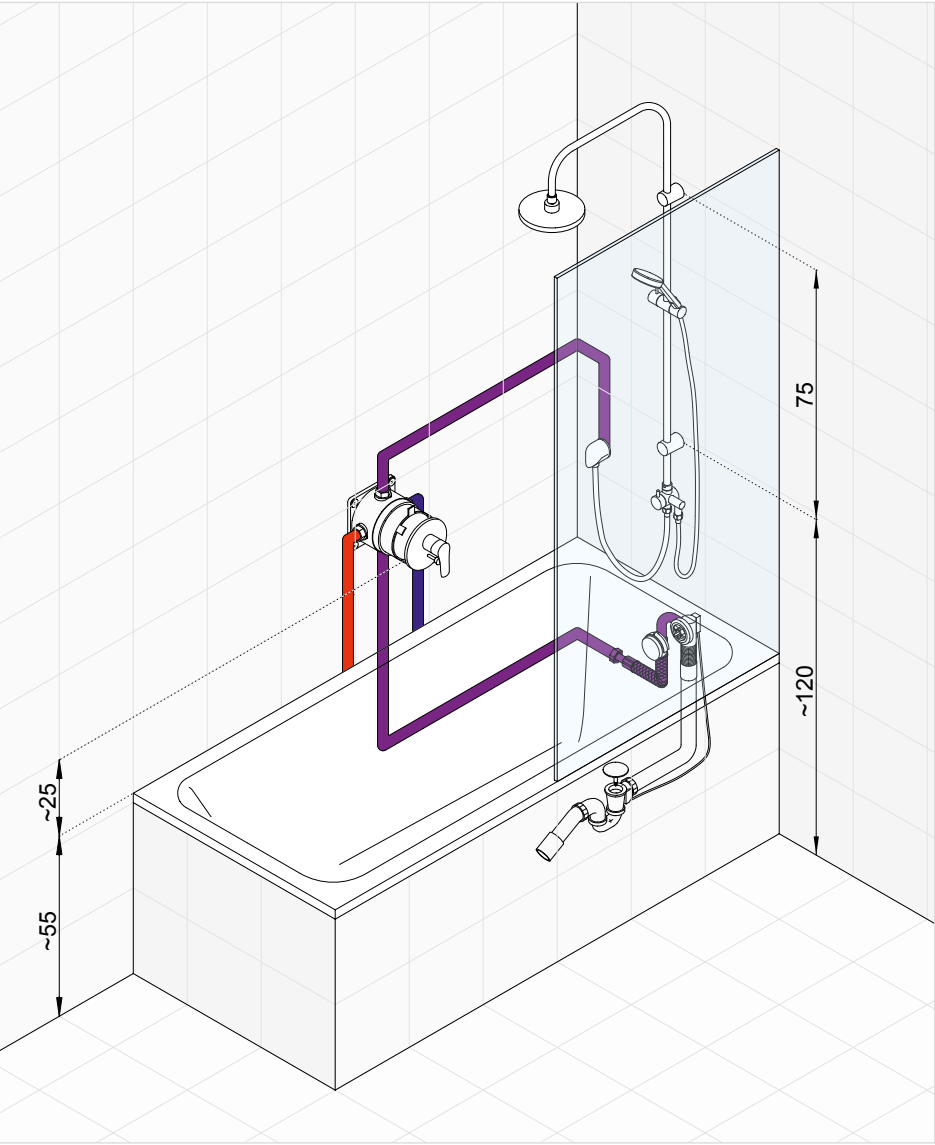
Vaňová a sprchová batéria umožňuje prepínať vodu medzi napúšťaním vane prepadom a KLUDI DUAL SHOWER SYSTÉMOM, ktorý umožňuje prepínať vodu medzi hlavovou a ručnou sprchou.
