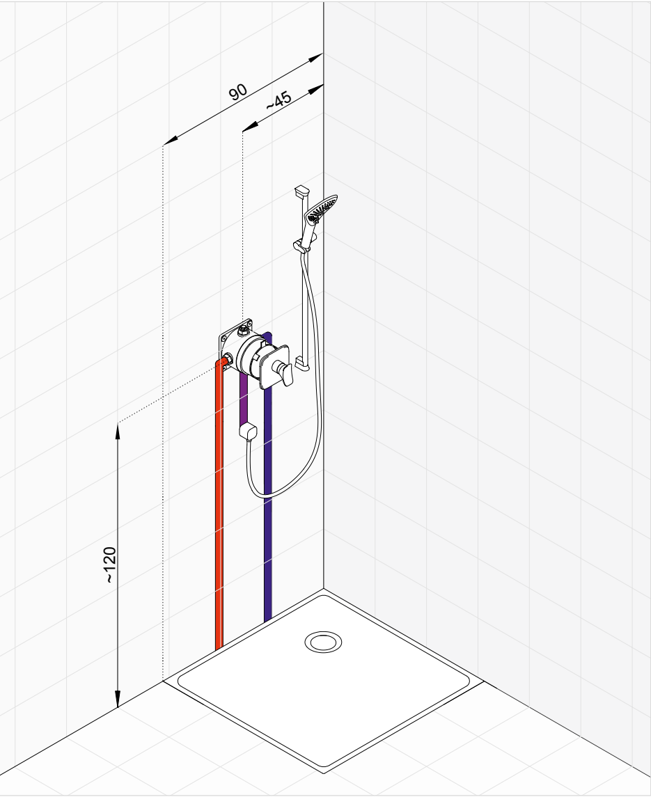
Klasický podomietkový rozvod k sprchovej súprave.
