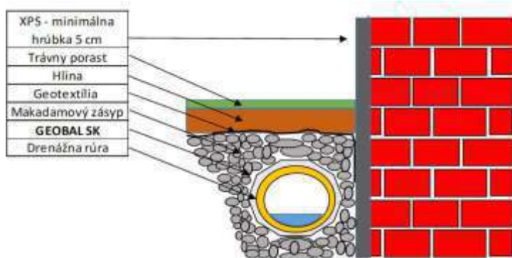
Izolácia základov
