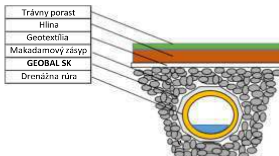
Lineárne odvodnenie
